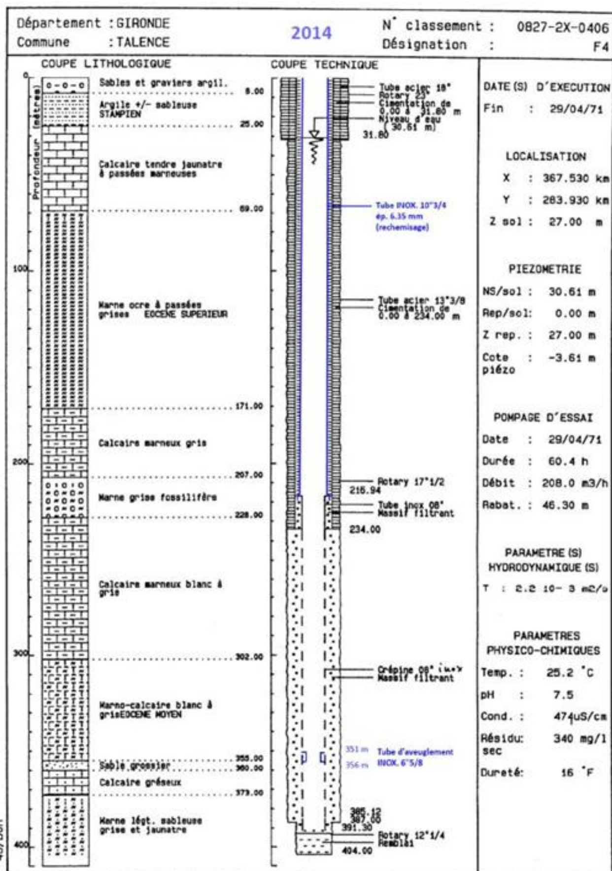
Figure 20 : Coupe technique du forage Lavardens – 2014 (source dossier d'enquête)
