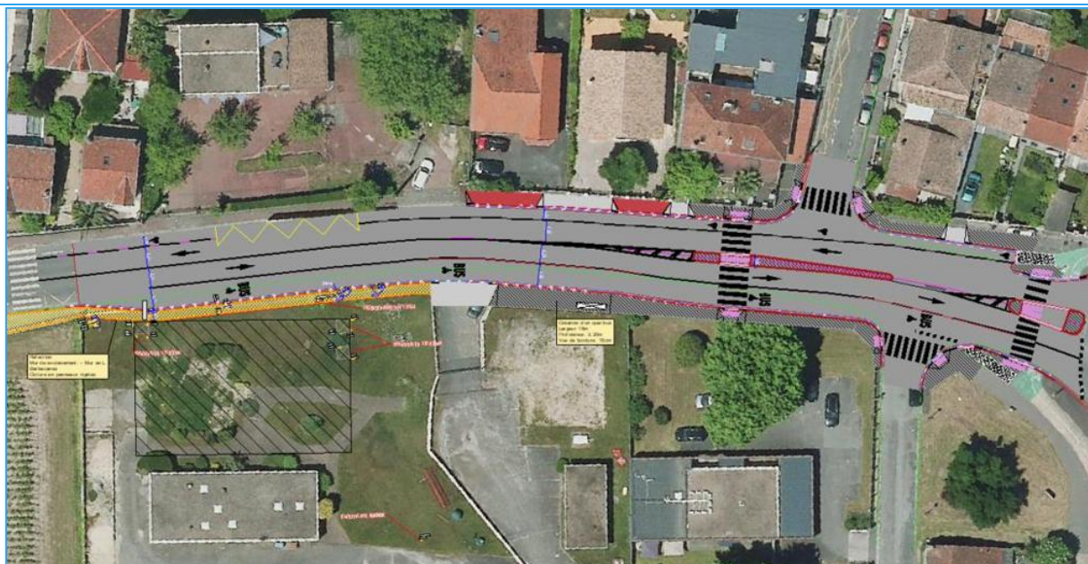
Figure 21 : Projet d'aménagement avec longueur linéaire totale de 150ml (source dossier d'enquête)
